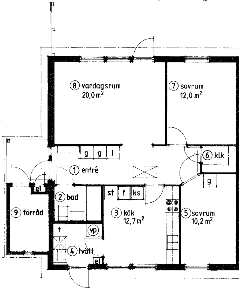
Entréplan, Av II. hus nr. 60 64 = 2 st Ah II. hus nr. 20 spegelvänt = 1 st
