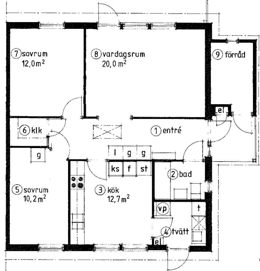
Entréplan, Ah I. hus nr. 27, 43, 52, 53 = 4 st Av I. Hus nr. 7, 21 , 36 , 46 86 spegelvänder = 5 st
